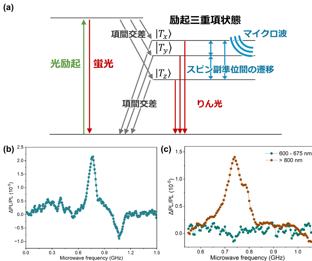
図 2: (a) 励起三重項を用いた ODMR 測定メカニズム。スピン選択的な項間交差により、励起三重項の三準位の間のポピュレーションに偏りが生じる。励起三重項間のエネルギー差に相当する周波数のマイクロ波を照射することでポピュレーションが変化し、蛍光やりん光の強度変化として読み出される。(b) ポルフィリン MOF のゼロ磁場 ODMR スペクトル。(c) 異なる波長で検出した際のゼロ磁場 ODMR スペクトル。
