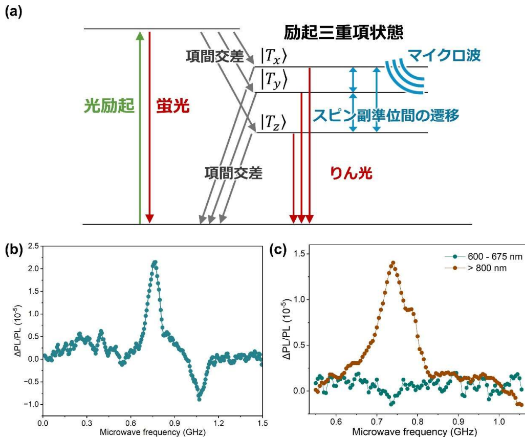
図 2: (a)励起三重項を用いた ODMR 測定のみカニズム。スピン選択的な項間交差により、励起三重項の三準位間のポピュレーションに偏りが生じる。励起三重項間のエネルギー差に相当する周波数のマイクロ波を照射することでポピュレーションが変化し、蛍光やりん光の強度変化として読み出される。(b)ポルフィリン MOF のゼロ磁場 ODMR スペクトル。(c)異なる波長で検出した際の ゼロ磁場 ODMR スペクトル。
