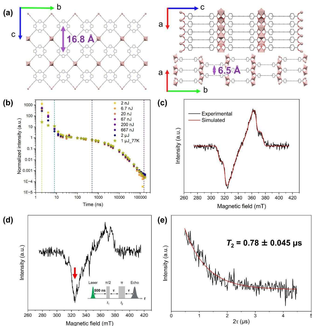
図 1: (a)本研究で用いたフリーベースポルフィリン MOF の結晶構造。(b) TRPL 測定によって得られた 720 nm における発光の減衰。(c) 過渡 ESR 測定によって得られた励起三重項の ESR スペクトル。(d) パルス ESR 測定によって得られた励起三重項の ESR スペクトル。インセット: 測定に使用されたパルスシーケンス。(e) 324.8 mT における励起三重項の信号の減衰とフィッティング曲線の時定数から得られたスピン—スピン緩和時間 T_2 。
