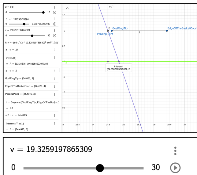
図 8 緑間選手がバスケットコート内でスリーポイントシュートを決めることができるボールの初速度の最大値
