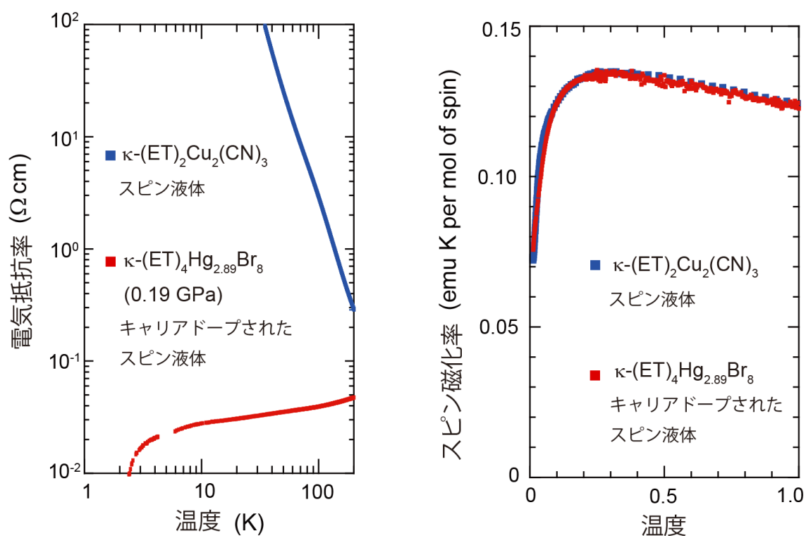
図3 スピン液体 \kappa\text{-(ET)}_2\text{Cu}_2(\text{CN})_3 とキャリアドーピングされたスピン液体 \kappa\text{-(ET)}_4\text{Hg}_{2.89}\text{Br}_8 の比較
