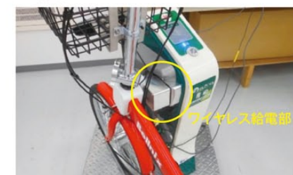
レンタル自転車のワイヤレス給電装置(2016年3月実証実験時)
